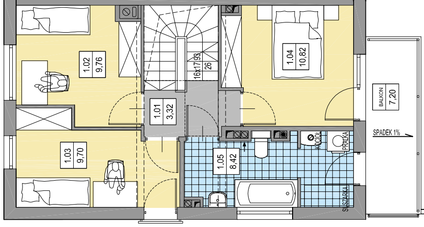
RZUT PIĘTRA
