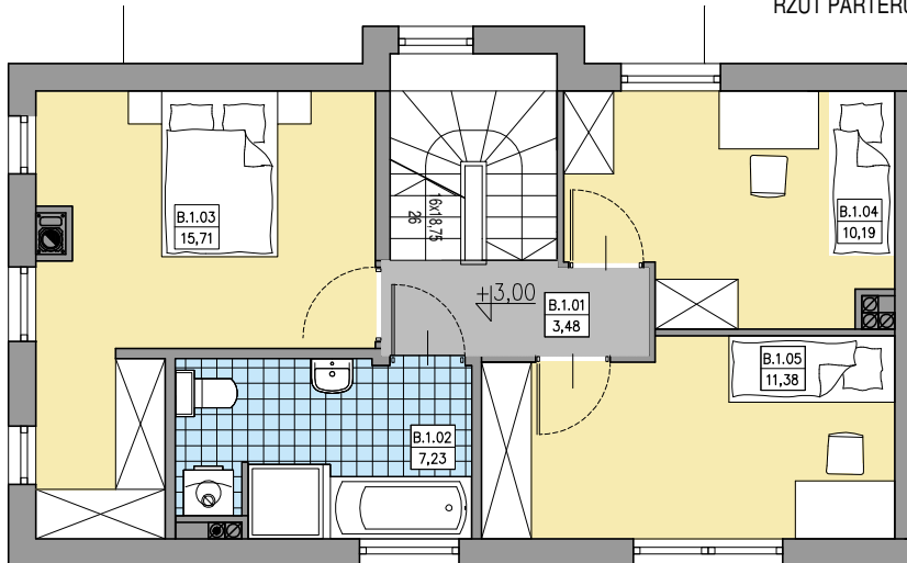
RZUT PIĘTRA
