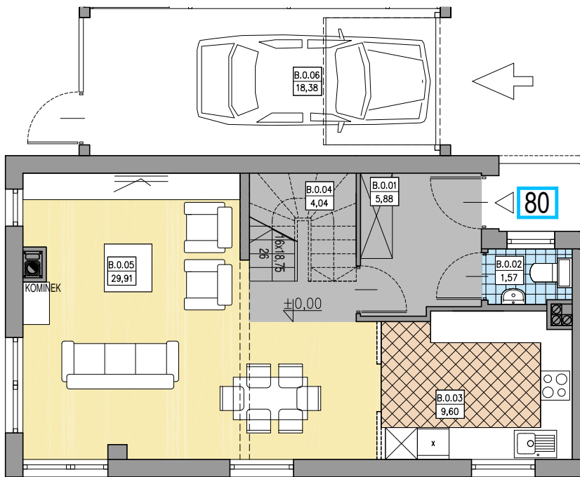
RZUT PARTERU
