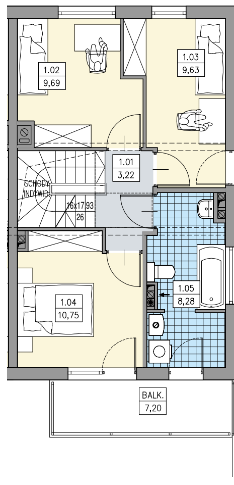
RZUT PIĘTRA
