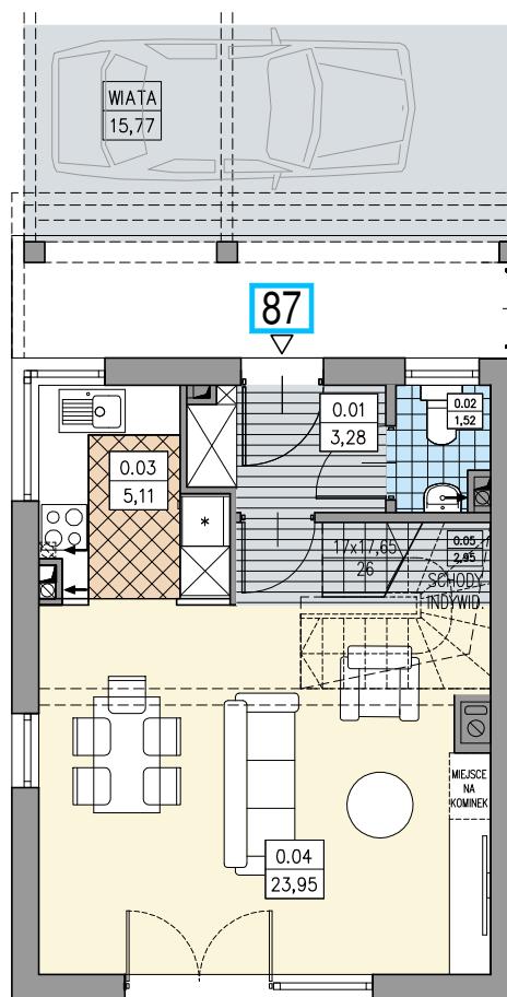
RZUT PARTERU
