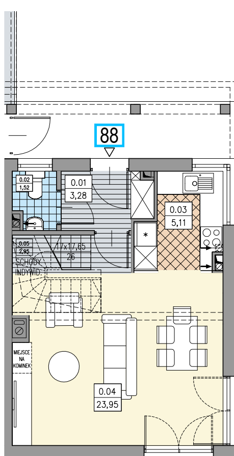
RZUT PARTERU
