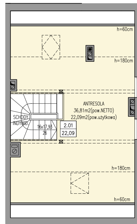
RZUT ANTRESOLI
